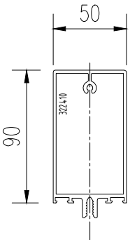
SECTION-A
