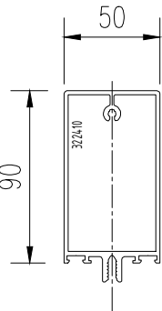
SECTION-A
