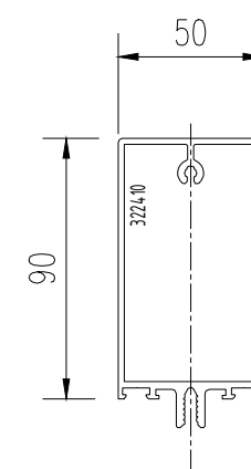
SECTION-A
